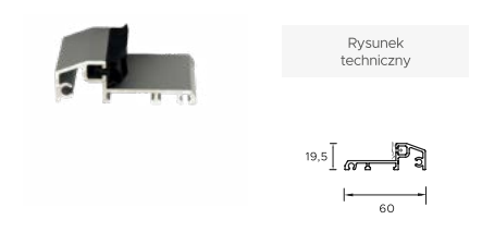
Próg Alu z uszczelką Premium
