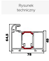
Ościeznica Termo Optimum
