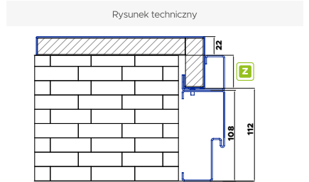
Przekrój łącznika kąтового Termo 90°
