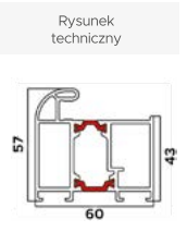
Ościeznica Termo Premium
