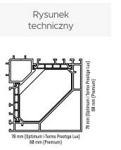
Przekrój łącznika kąтового Termo 90°
